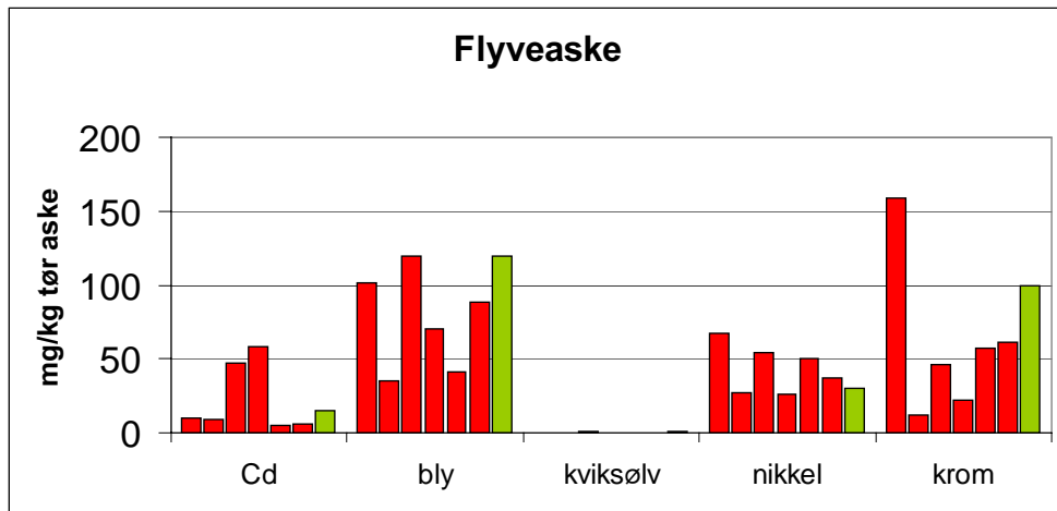
Figur 1 Indhold af tungmetaller i flyveaske og afskæringsværdier (højre søjle, lys) for indhold af tungmetaller, jf. bioaskebekendtgørelsen.
