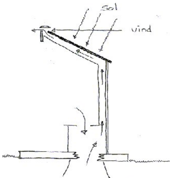
Figur 1. Solmultens princip. De mørke plader på taget skaber varme og dermed en luftstrøm, og vindfanget øverst på taget bidrager til, at trækket øges gennem et undertryk!
