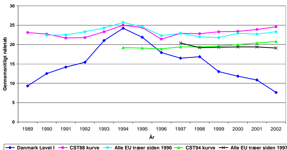
Figur 11. Det gennemsnitlige nåletab for rødgran siden overvågningens start i 1989. Udviklingen for Danmark bygger på samtlige overvågningspunkter, dvs. både EU punkter og nationale punkter. De europæiske udviklingskurver bygger på to forskellige tidsserier, som udgør en mindre del af samtlige punkter. CST 94 repræsenterer f.eks. 46 % af alle punkter.
